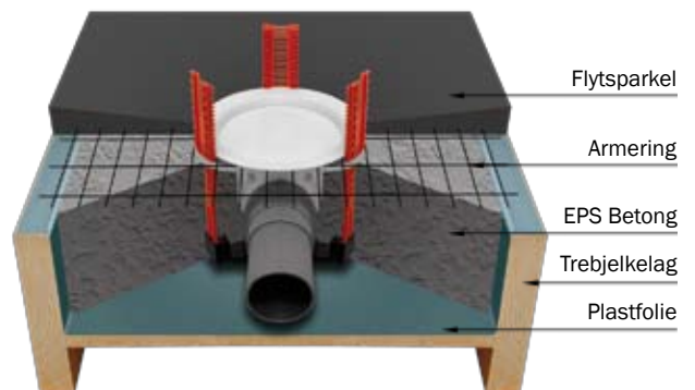
Eksempel på montering av sluk i trebjelkelag med JAFØ Innstøpningsstativ
